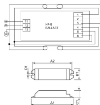
Specifikationer Philips HF-E 236 TL-D II 220-240V 50/60Hz for 2x36W
